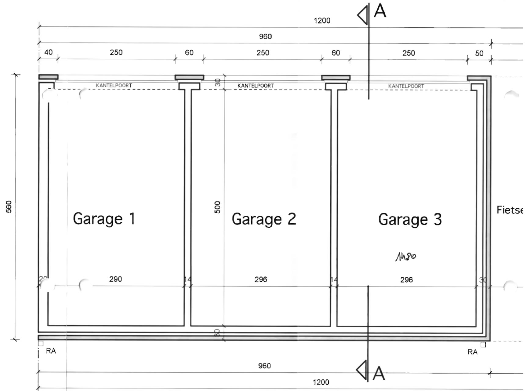
Grondplan
