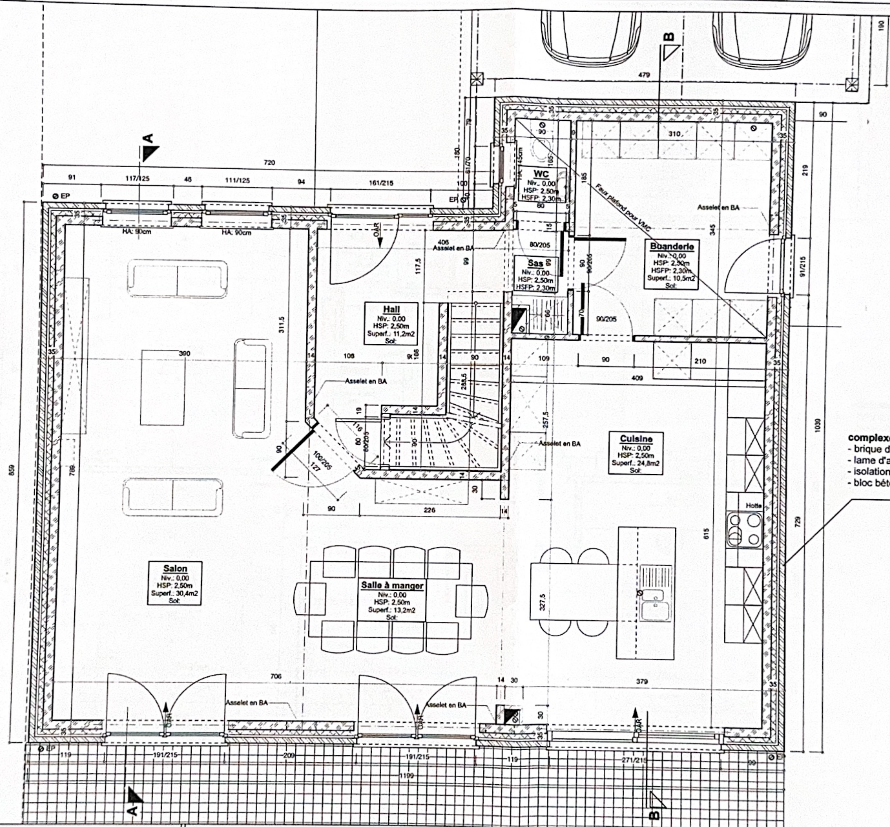
PLAN REZ-DE-CHAUSSEE
