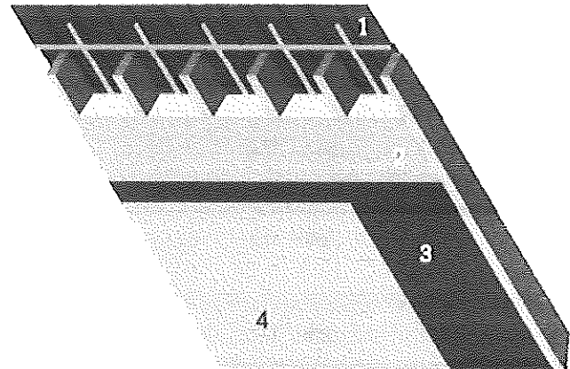
1. Onderdak | 2. Isolatie | 3. Dampscherm | 4. binnenaferking
