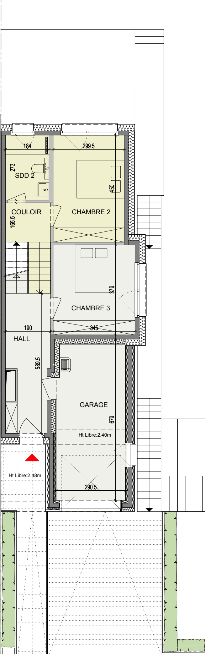
REZ-DE-CHAUSSEE MEZ RDC 1:100
