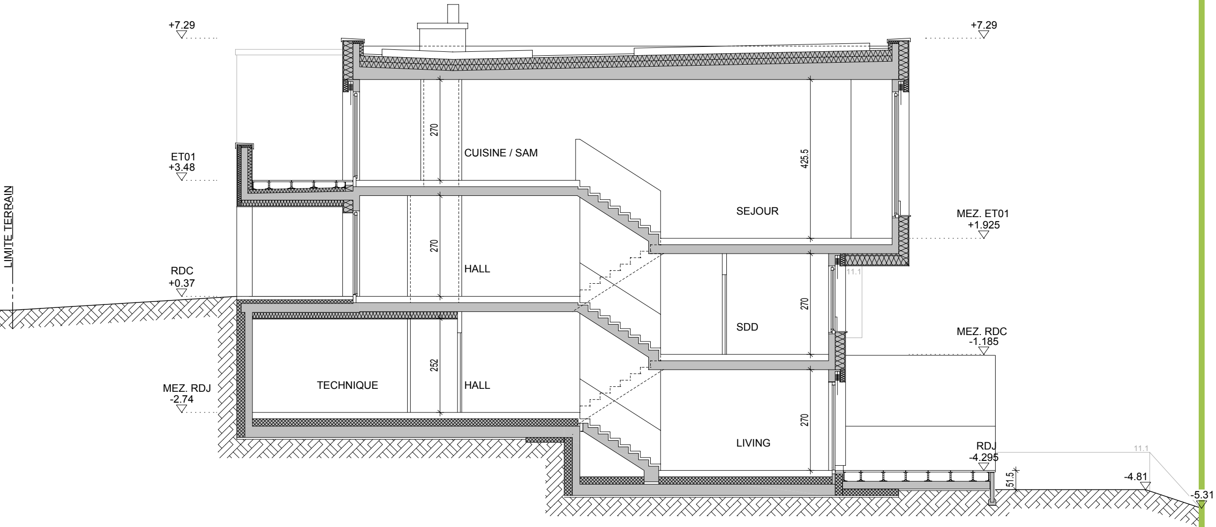
COUPE 1:100
