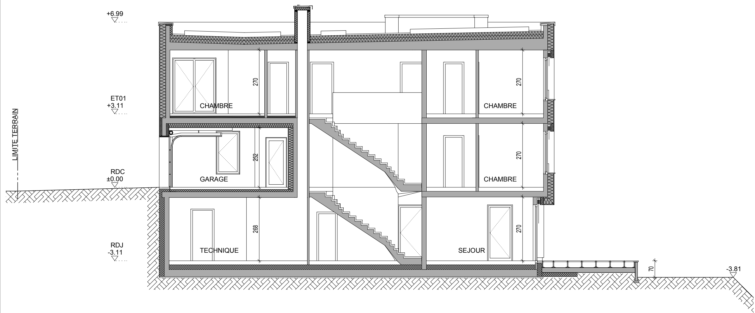
COUPE 1:100
