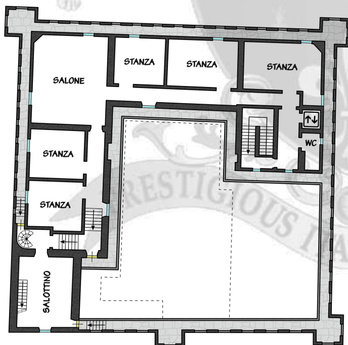
PIANO SECONDO
